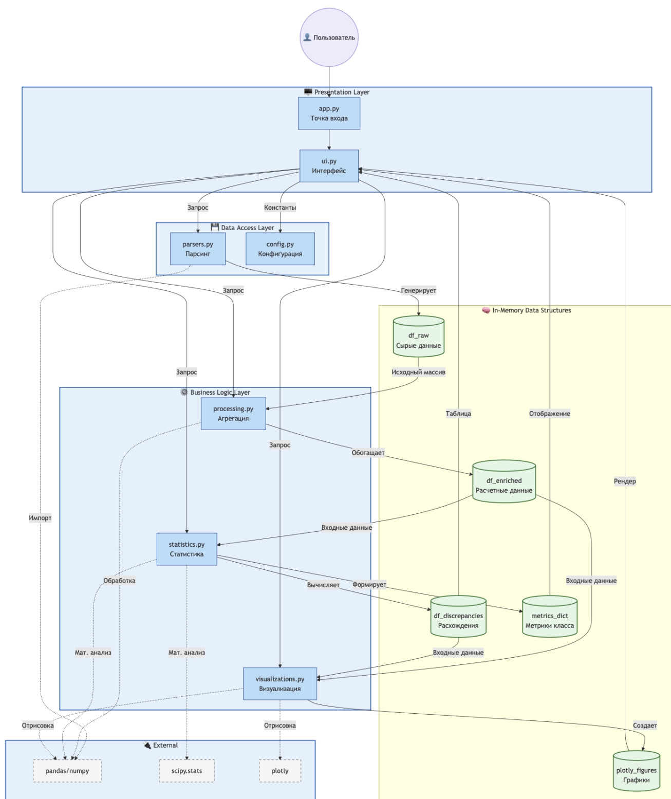
Рисунок 3 – Архитектура решения (Solution)
