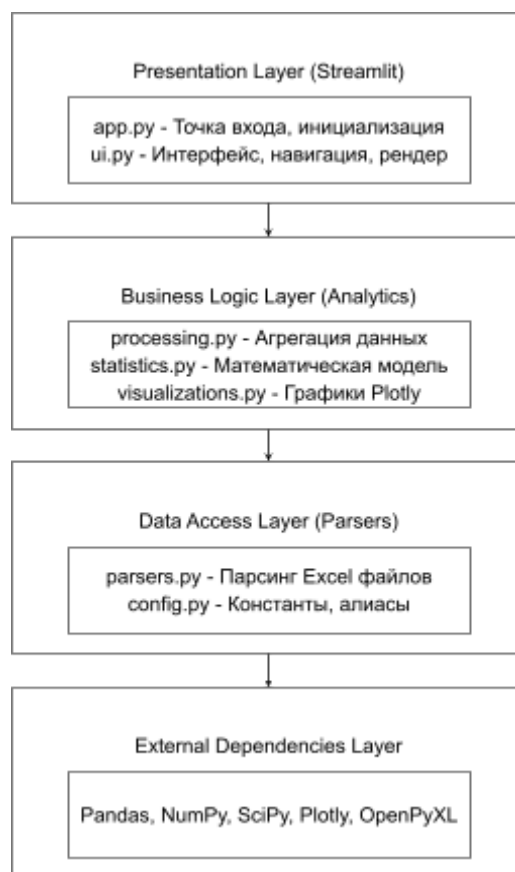
Рисунок 2 – Уровни компонентов программного средства
